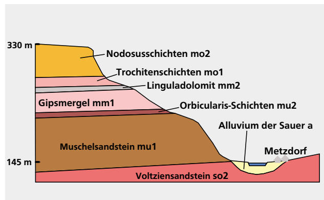
Geologischer Querschnitt durch das Untere Sauerthal, 2-fach überhöhte Darstellung
